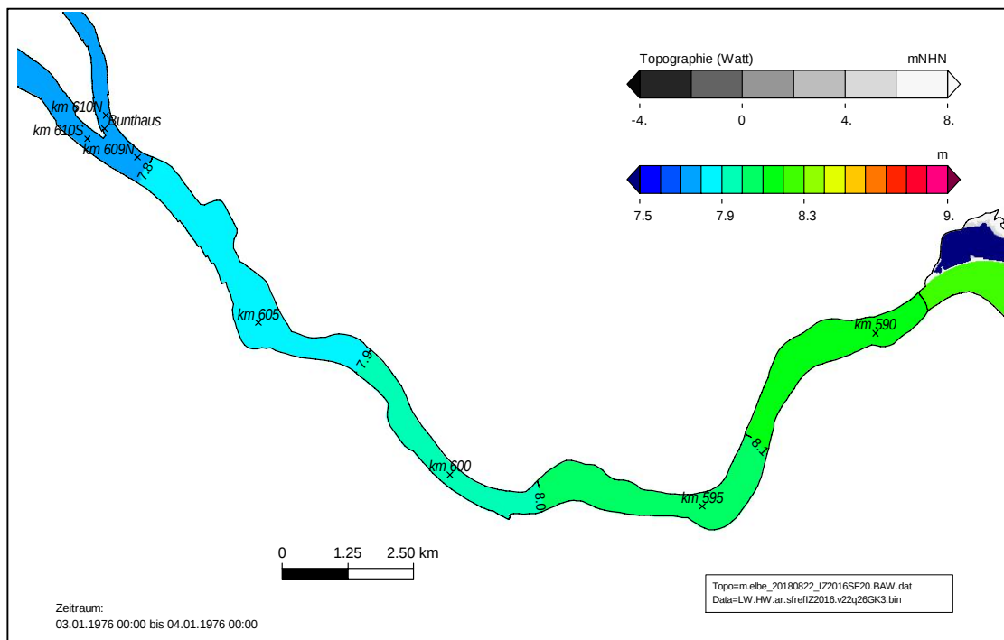
Bild 35: SFREF (IJ2016): Sturmflutscheitelwasserstand HW für das Sturmflutszenario SFREFQ2600 im Teilgebiet Ost zwischen Bunthaus und Geesthacht. Eine Farbstufe entspricht einem Unterschied im HW von 10 cm.
