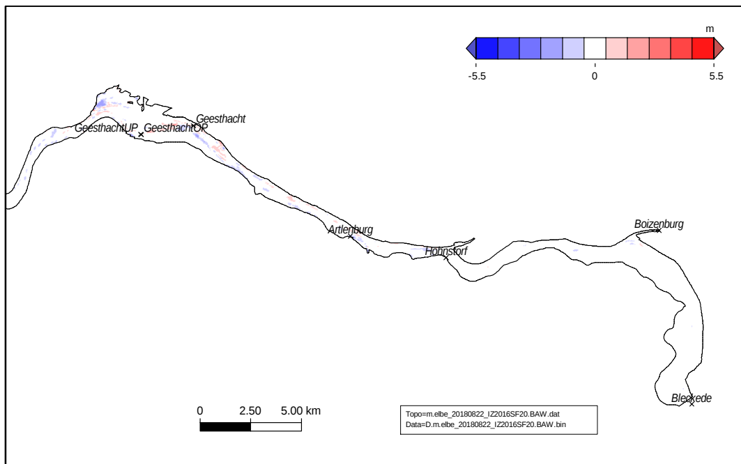
Bild 15: Teilgebiet Mittelelbe: Änderung der Topographie des numerischen Modells des Elbeästuares der BAW für Sturmflutuntersuchungen IZ2016 (2016) im Vergleich zu PIZ02 (2010). Eine Farbstufe entspricht einer Tiefenänderung von 100 cm. In den weiß dargestellten Gebieten ändert sich die Topographie um weniger als \pm 50 cm. In den blau dargestellten Bereichen ist die Topographie 2016 tiefer als 2010. In den rot dargestellten Bereichen ist die Topographie 2016 flacher als 2010.
