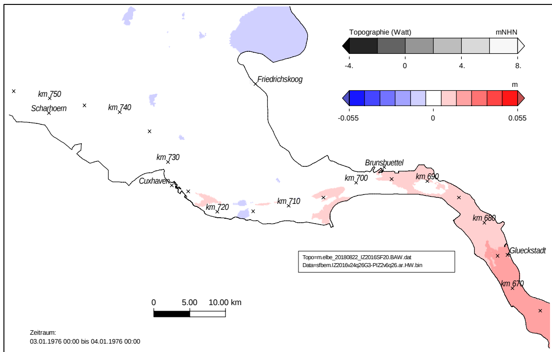
Bild 27: SFBEM (IZ2016) – SFBEM (PIZ02): Änderung des Sturmflutscheitelwasserstandes HW für das Sturmflutszenario SFBEMQ2600 im Teilgebiet West. Eine Farbstufe entspricht einem Unterschied im HW von 1 cm. In den weiß dargestellten Gebieten ändert sich das HW um weniger als \pm 0,5 cm.
