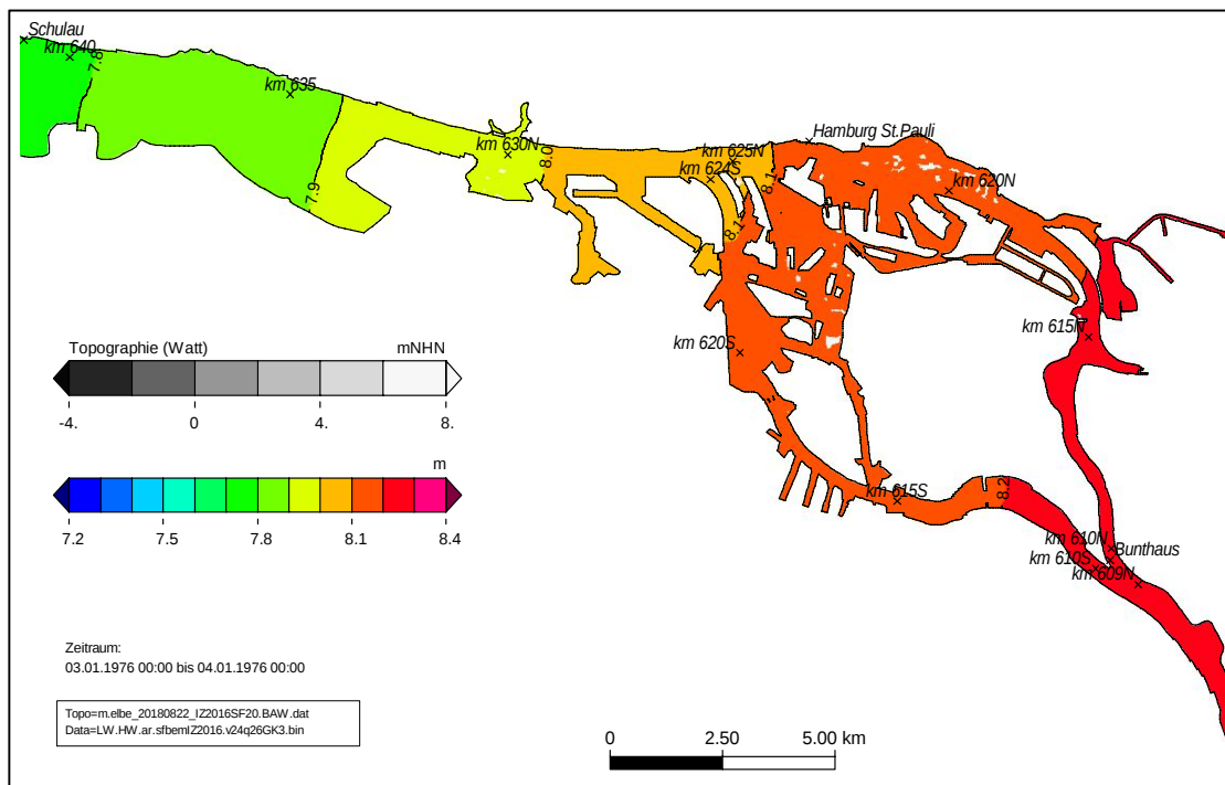
Bild 32: SFBEM (IJ2016): Sturmflutscheitelwasserstand HW für das Sturmflutszenario SFBEMQ2600 im Teilgebiet Hamburg zwischen Schulau und Bunthaus. Eine Farbstufe entspricht einem Unterschied im HW von 10 cm.
