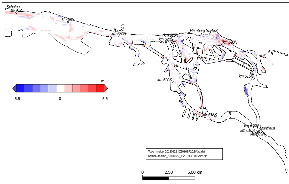
Bild 9: Teilgebiet Hafen: Änderung der Topographie des numerischen Modells des Elbeästuares der BAW für Sturmflutuntersuchungen IZ2016 (2016) im Vergleich zu PIZ02 (2010). Eine Farbstufe entspricht einer Tiefenänderung von 100 cm. In den weiß dargestellten Gebieten ändert sich die Topographie um weniger als \pm 50 cm. In den blau dargestellten Bereichen ist die Topographie 2016 tiefer als 2010. In den rot dargestellten Bereichen ist die Topographie 2016 flacher als 2010.
