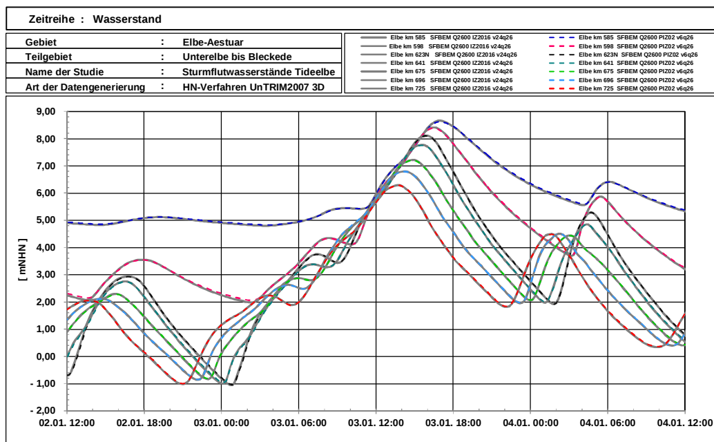
Bild 19: SFBEMQ2600: Wasserstandsentwicklung entlang der Elbe bei Cuxhaven (Elbe – km 725; rot), Brunsbüttel (Elbe – km 696, cyan), Glückstadt (Elbe – km 675, grün), Schulan (Elbe – km 641, dunkelgrün), Hamburg St. Pauli (Elbe – km 623N, schwarz), Zollenspieker (Elbe – km 598, magenta) und Geesthacht (Elbe – km 585, blau) (Datum ohne Bedeutung) in der Topographie 2010 (PIZ02) gestrichelt in Farbe und in der Topographie 2016 (IZ2016) durchgezogen in Grau.
