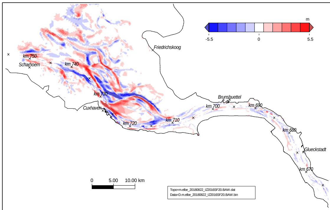
Bild 6: Teilgebiet West: Änderung der Topographie des numerischen Modells des Elbeästuares der BAW für Sturmflutuntersuchungen IZ2016 (2016) im Vergleich zu PIZ02 (2010). Eine Farbstufe entspricht einer Tiefenänderung von 100 cm. In den weiß dargestellten Gebieten ändert sich die Topographie um weniger als \pm 50 cm. In den blau dargestellten Bereichen ist die Topographie 2016 tiefer als 2010. In den rot dargestellten Bereichen ist die Topographie 2016 flacher als 2010.
