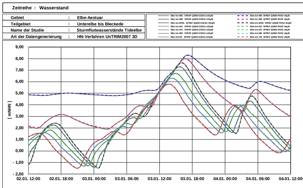
Bild 18: SFREFQ2600: Wasserstandsentwicklung entlang der Elbe bei Cuxhaven (Elbe – km 725, rot), Brunsbüttel (Elbe – km 696, cyan), Glückstadt (Elbe – km 675, grün), Schulan (Elbe – km 641, dunkelgrün), Hamburg St. Pauli (Elbe – km 623N, schwarz), Zollenspieker (Elbe – km 598, magenta) und Geesthacht (Elbe – km 585, blau) (Datum ohne Bedeutung) in der Topographie 2010 (PIZ02) gestrichelt in Farbe und in der Topographie 2016 (IZ2016) durchgezogen in Grau.
