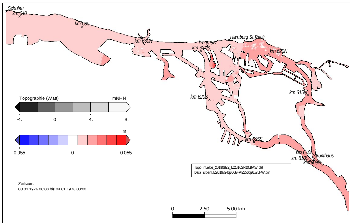
Bild 33: SFBEM (IZ2016) – SFBEM (PIZ02): Änderung des Sturmflutscheitelwasserstandes HW für das Sturmflutszenario SFBEMQ2600 im Teilgebiet Hafen. Eine Farbstufe entspricht einem Unterschied im HW von 1 cm. In den weiß dargestellten Gebieten ändert sich das HW um weniger als \pm 0,5 cm.
